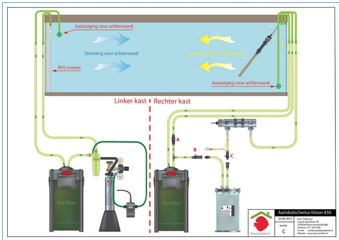
Bij dit ontwerp is de 3D achterwand niet afgebeeld. De uitvoer van de potfilters, nitraat/fosfaatfilter en UV lamp zitten achter de 3D achterwand, via een RVS rooster (links) kan het gefilterde water naar het aquarium stromen. Door deze constructie zijn de leidingen en de verwarming netjes weggewerkt en er is een constante stroming (gele pijlen) achter de achterwand. De waterinlaat naar de potfilters zit aan de voorkant van de 3D achterwand (linksboven en rechtsonder) Met de kranen A, B en C kan je de doorvoersnelheid naar de nitraat/fosfaatfilter en UV lamp regelen. Alle filters kunnen eenvoudig losgekoppeld worden voor het schoonmaken van de filters.
