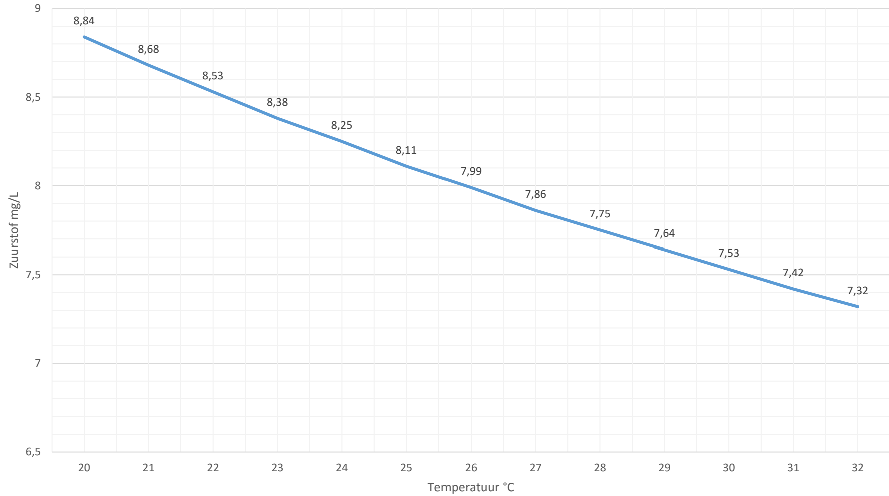
Zuurstof (O 2 ) verzadigingswaarde in water bij verschillende de temperaturen
