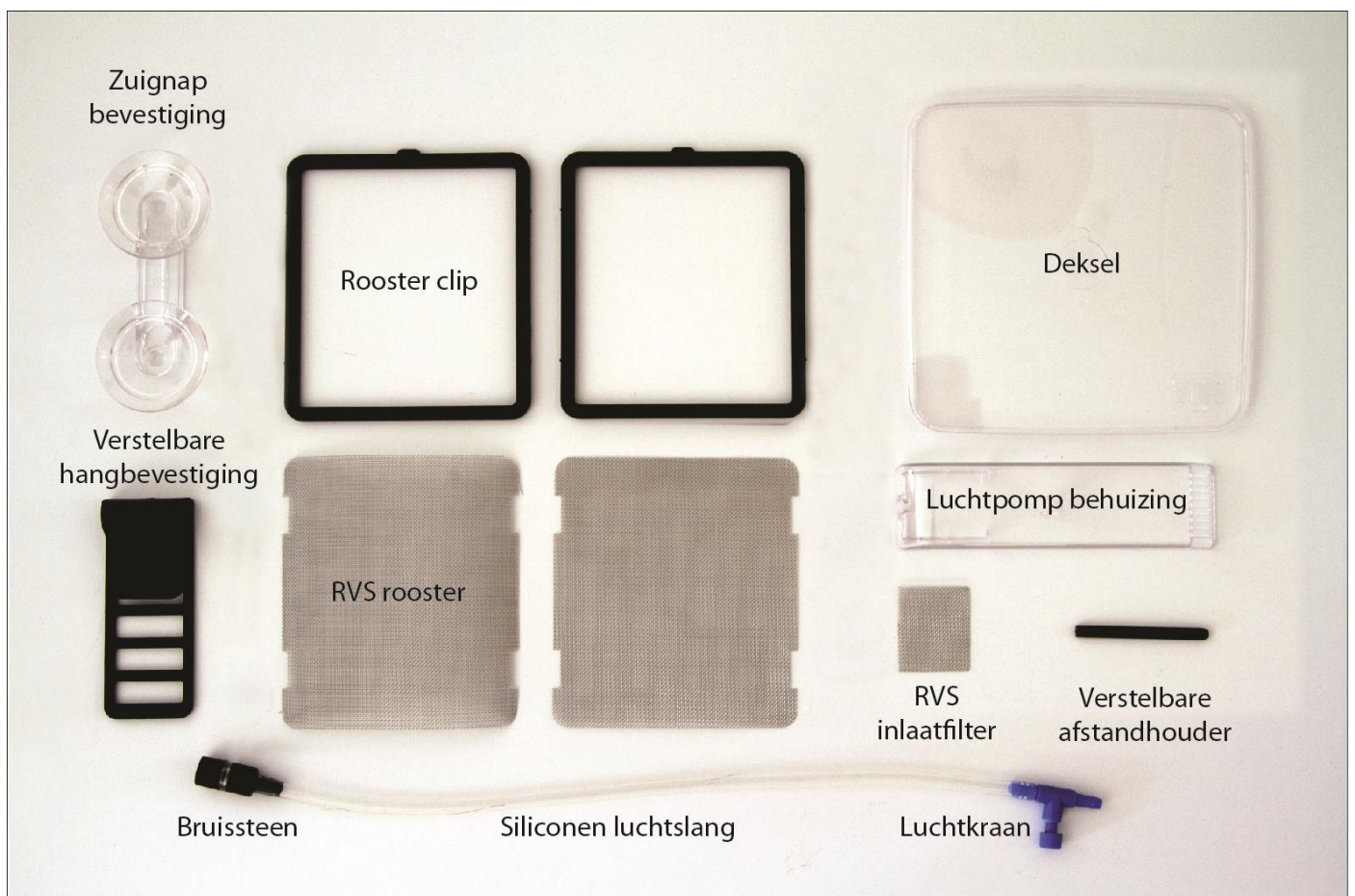
Onderdelenoverzicht (exclusief kweekbakje)
