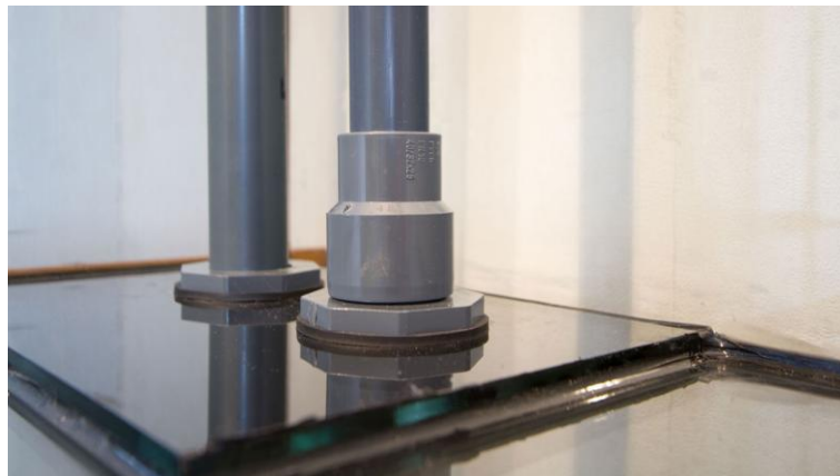
De overlooppijp en de aanvoerpijp zijn gemonteerd op een extra glasplaat. Dit voorkomt een mogelijke overbelasting van de aquariumbodem. De aanvoerleiding heeft een kleinere diameter dan de overlooppijp.
