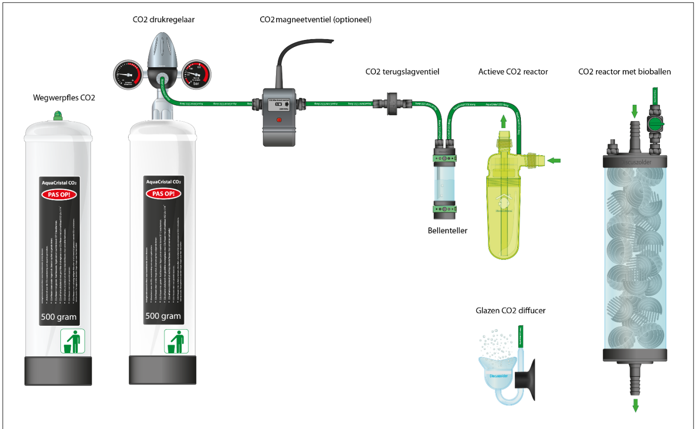
Een voorbeeld van een CO2 bemestingsysteem met wegwerpflessen.
