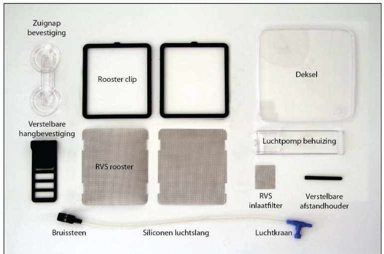
Onderdelenoverzicht (exclusief kweekbakje)
