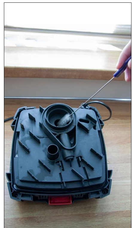
Met potfilter borsteltje kan je de rotor behuizing gemakkelijk schoonmaken.
